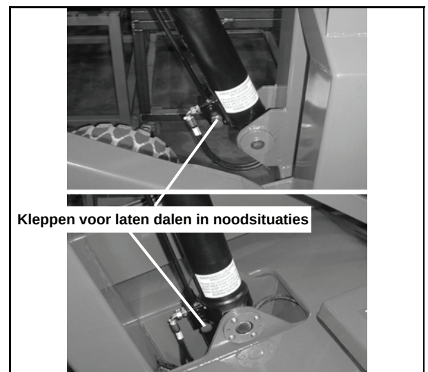
Afbeelding 3: Klep voor het laten dalen in noodsituaties
